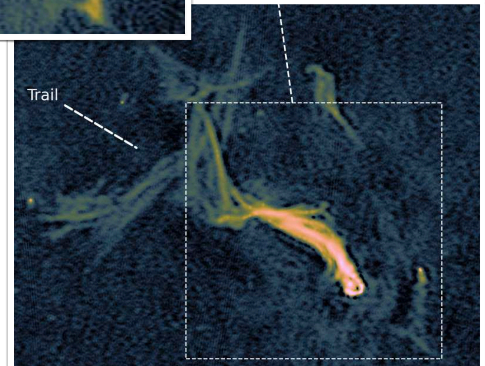
0.3" LOFAR VLBI De Rubeis + 2025, 2026
