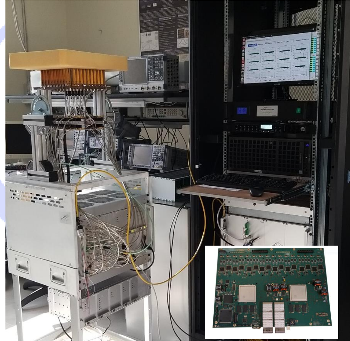
Sistema beamformer per PAF PHAROS2
