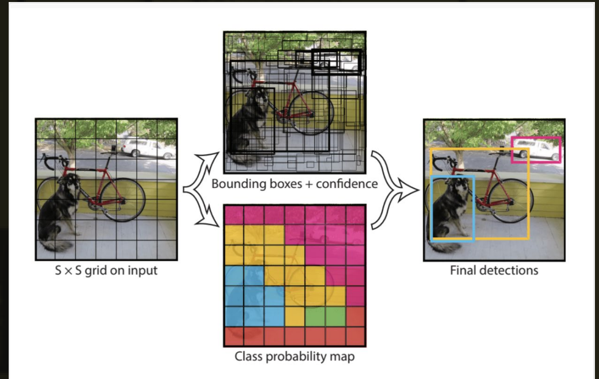
YOLO-V5
